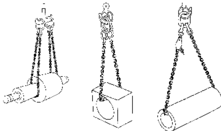
Obrázek 4 : Vázání podvlečením
